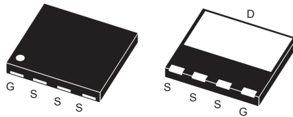
DFN8*8
