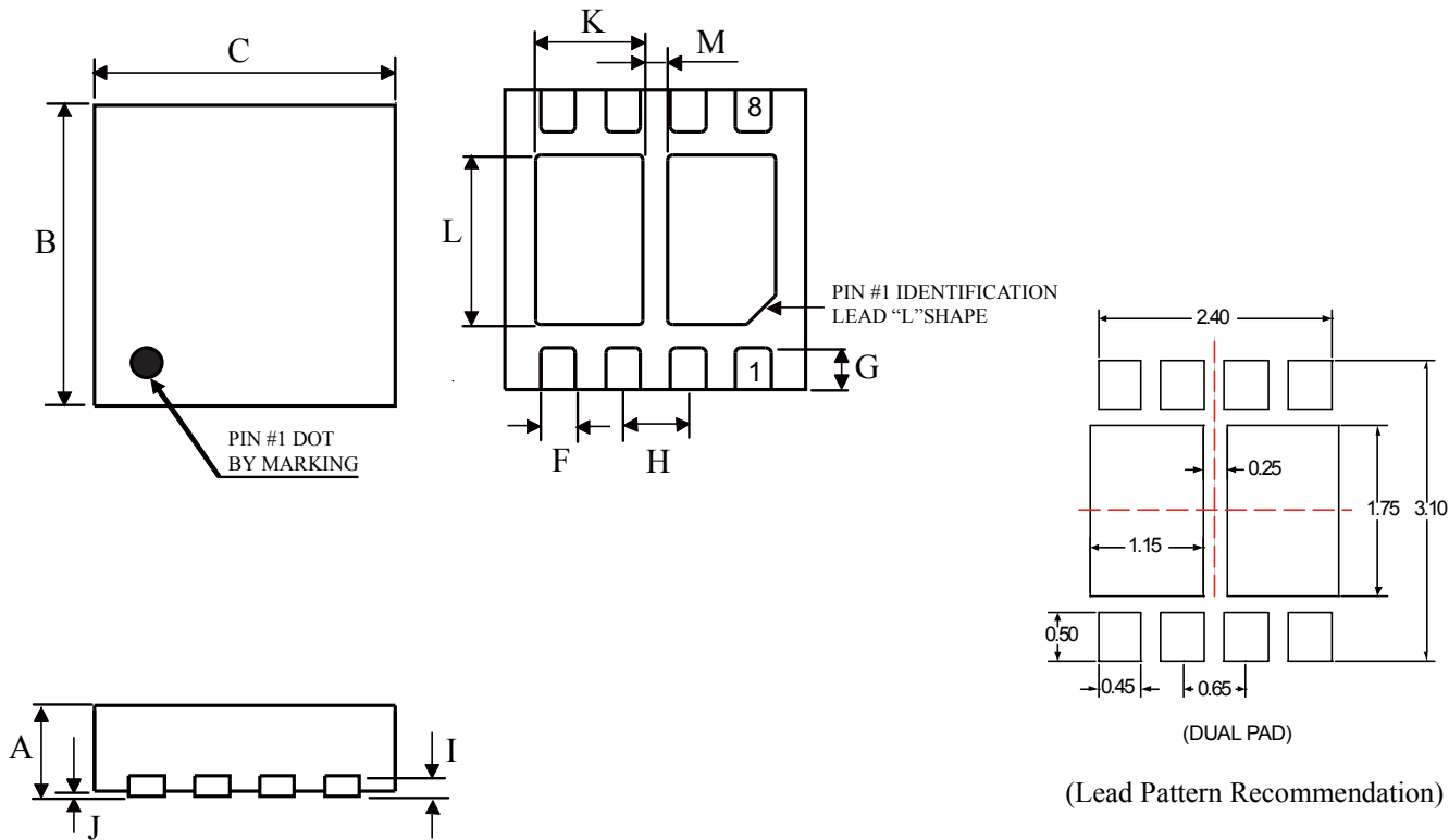
DUAL PAD 尺寸圖
