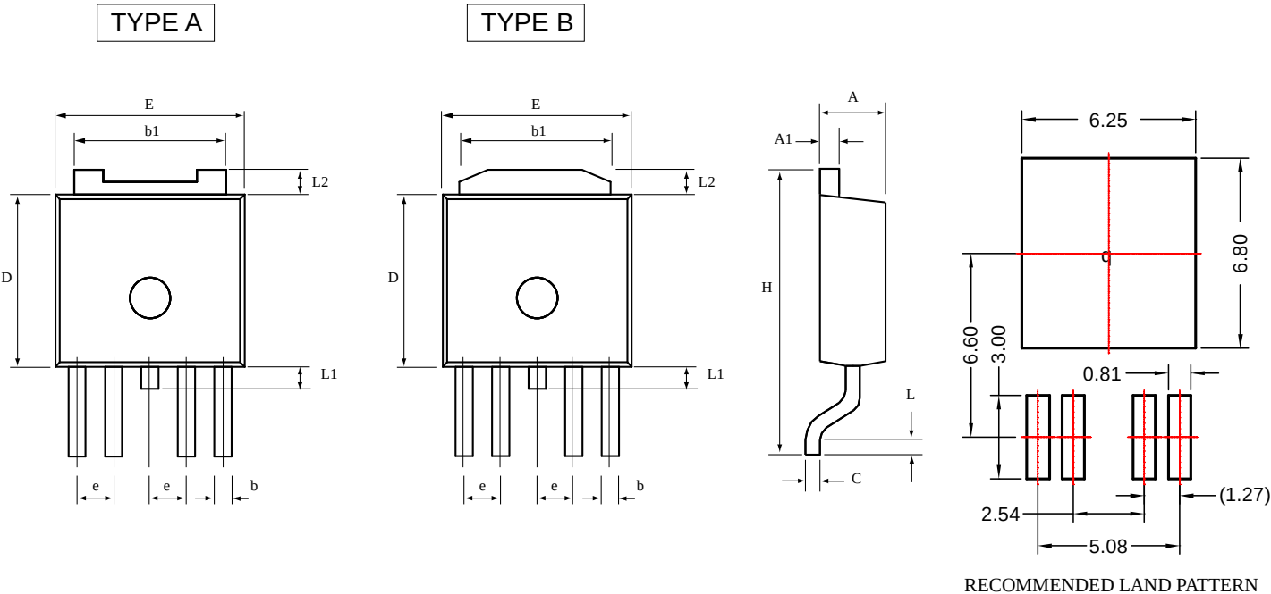
TO-252-4L 尺寸圖
