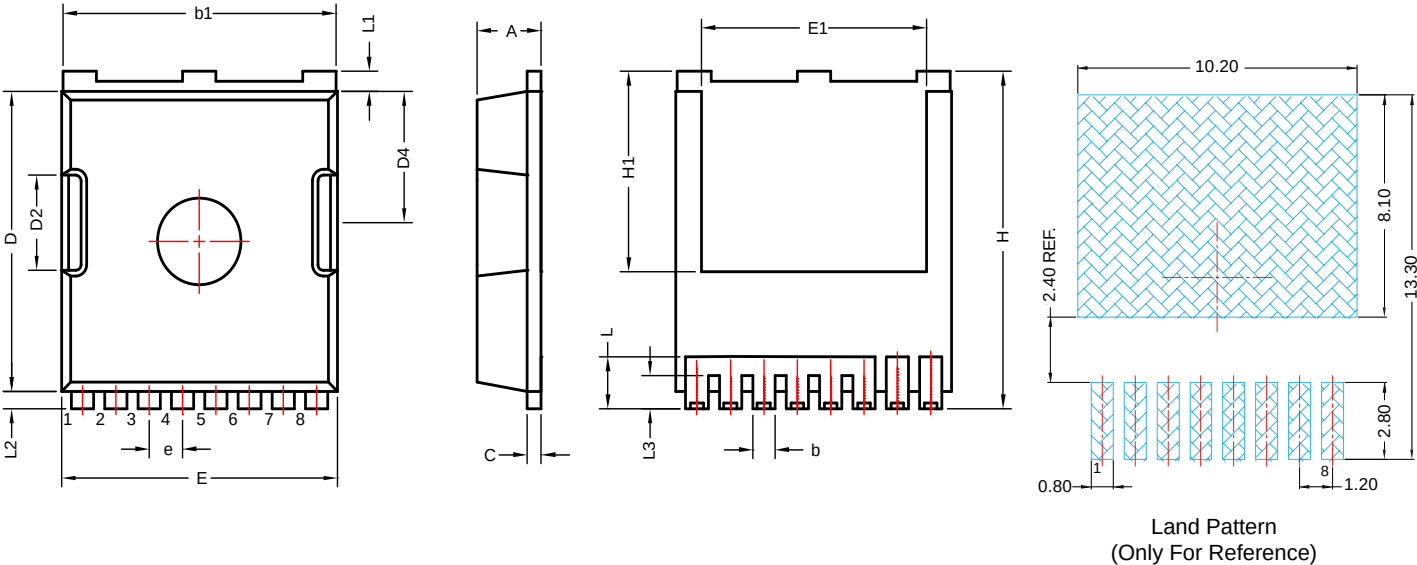
1.2 TOLL (Kelvin Source) 產品尺寸圖
