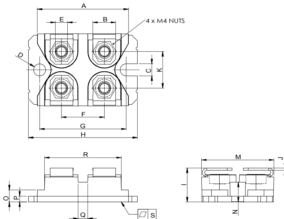
SOT-227 產品外觀尺寸圖 (Product Outline Dimension)
