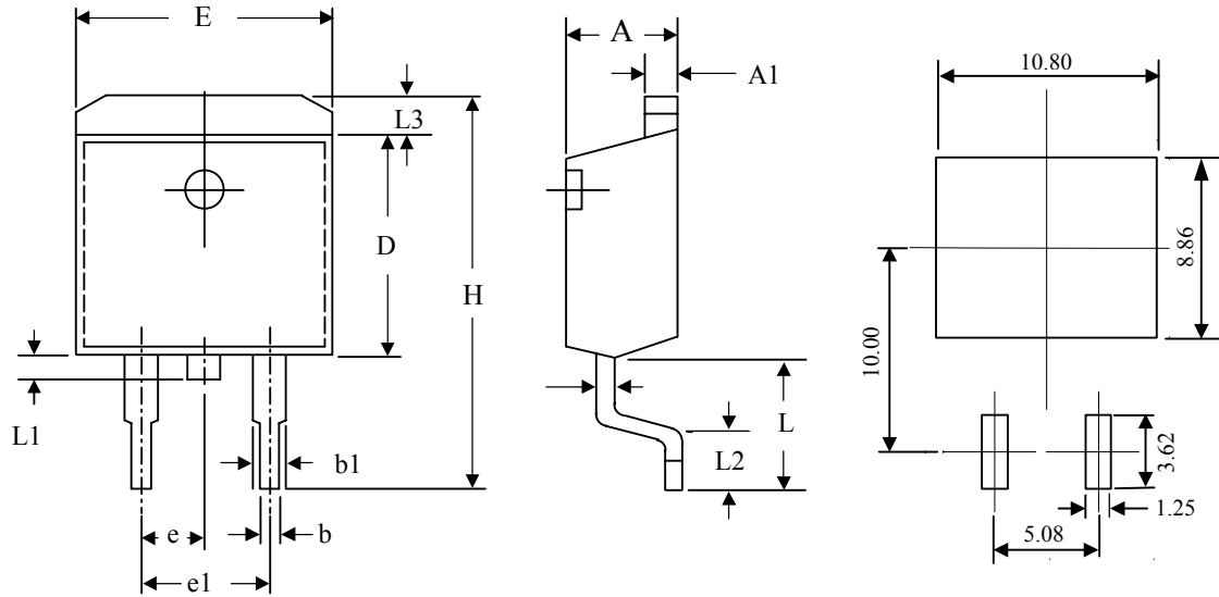
TO-263 產品外觀尺寸圖 (Product Outline Dimension)
