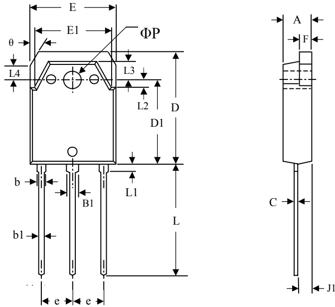
TO-3P 產品外觀尺寸圖 (Product Outline Dimension)
