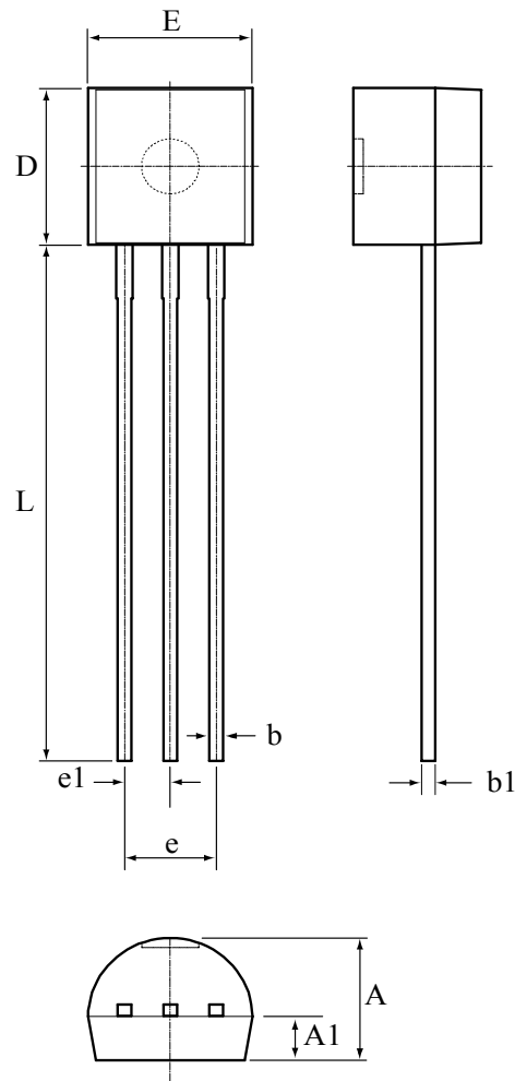
TO-92 產品外觀尺寸圖 (Product Outline Dimension)
