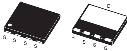
DFN8*8
