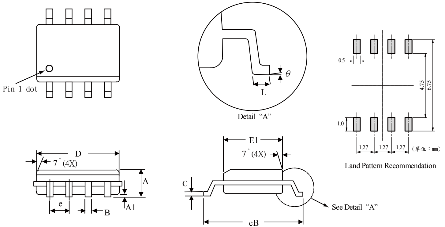
SOP-8 產品外觀尺寸圖 (Product Outline Dimension)
