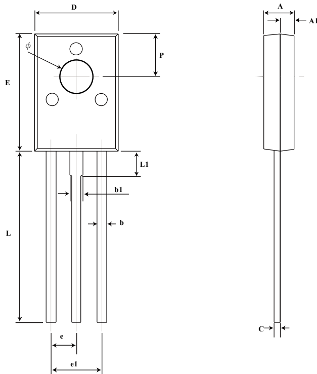
TO-126F 產品外觀尺寸圖 (Product Outline Dimension)
