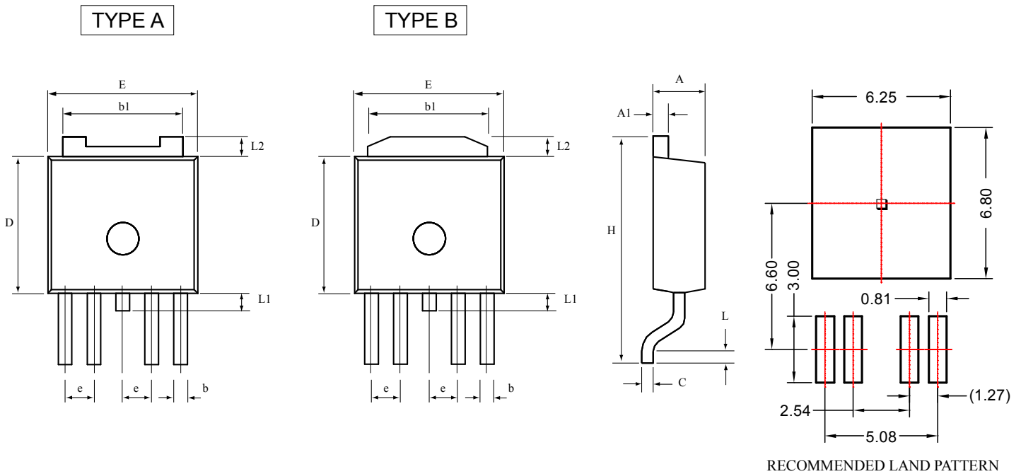
TO-252-4L 尺寸圖
