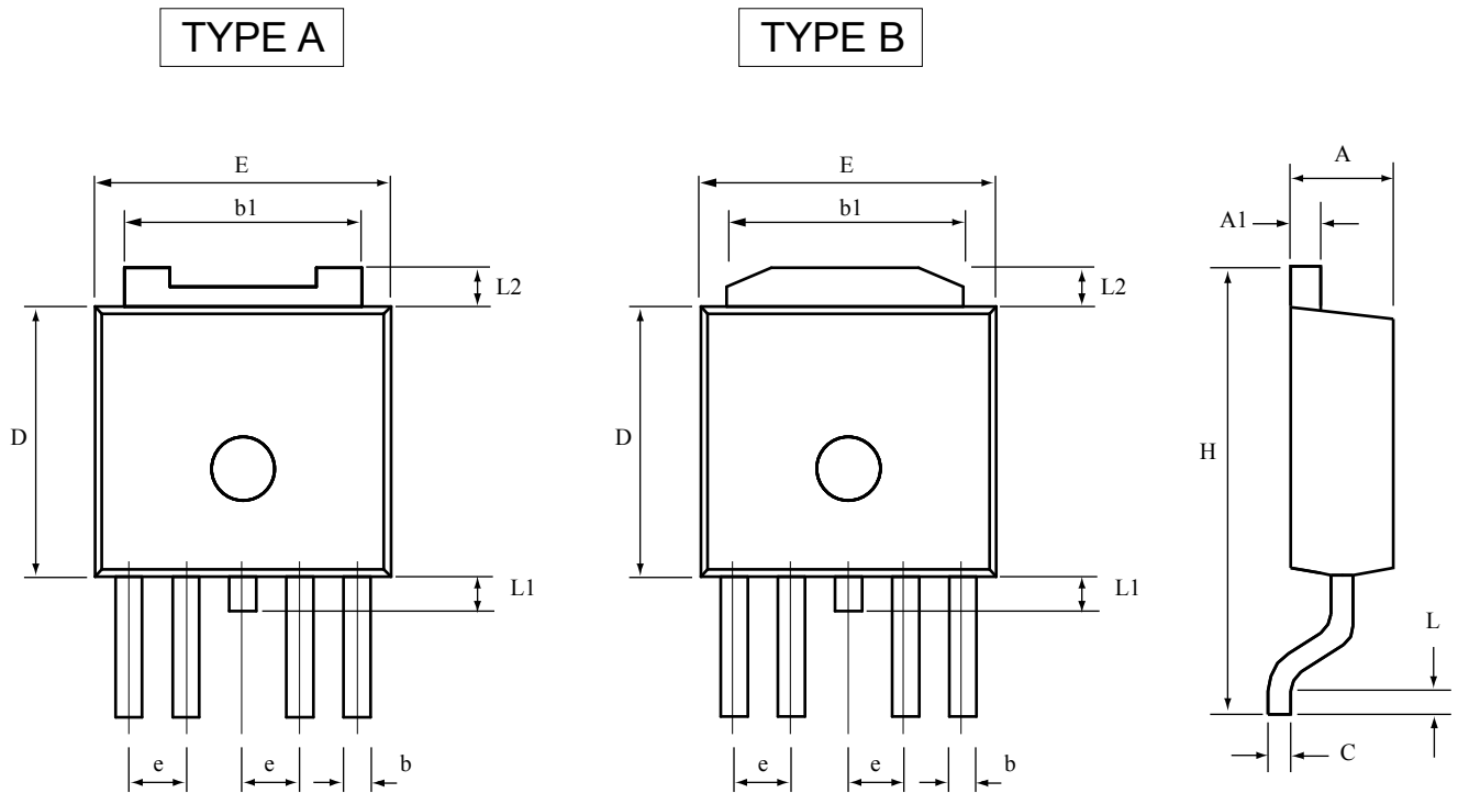
TO-252-4L 尺寸圖
